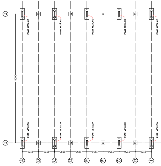
PLANTA DE LOCAÇÃO ESC: 1/100
