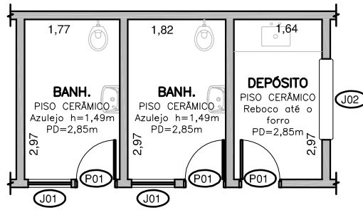
BANHEIROS E DEPÓSITO- SITUAÇÃO ATUAL 1:100
