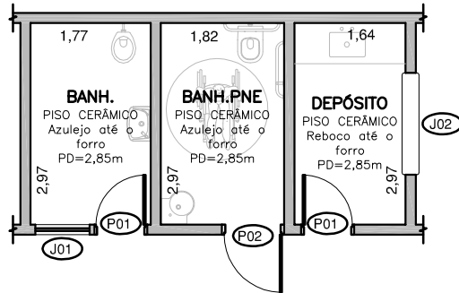
BANHEIROS E DEPÓSITO- PÓS REFORMA 1:100
