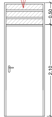
VISTA P02 1:50
