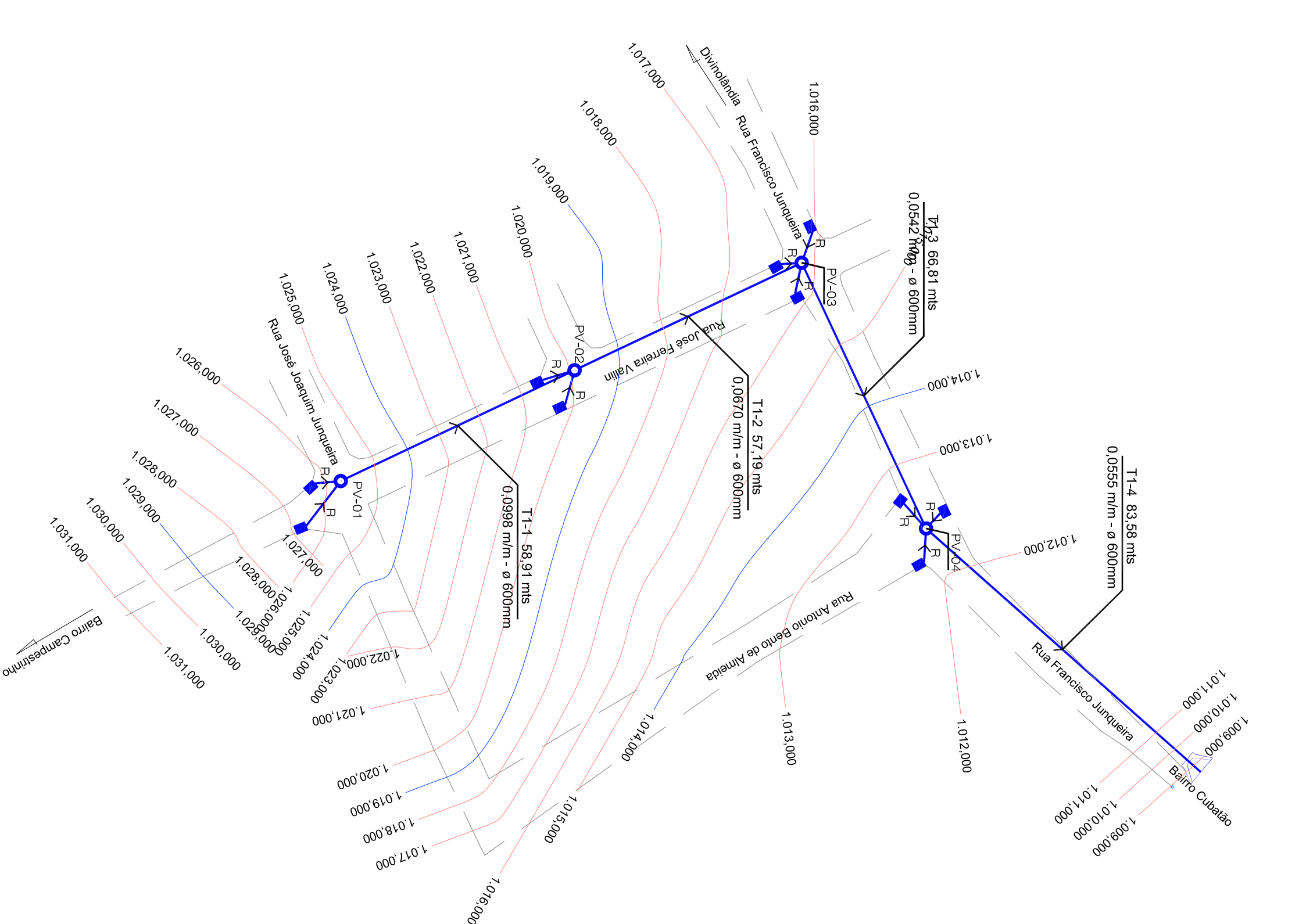
PLANTA BAIXA - RUAS DO BAIRRO RIBEIRÃO DO SANTO ANTÔNIO ESC: 1:1000
