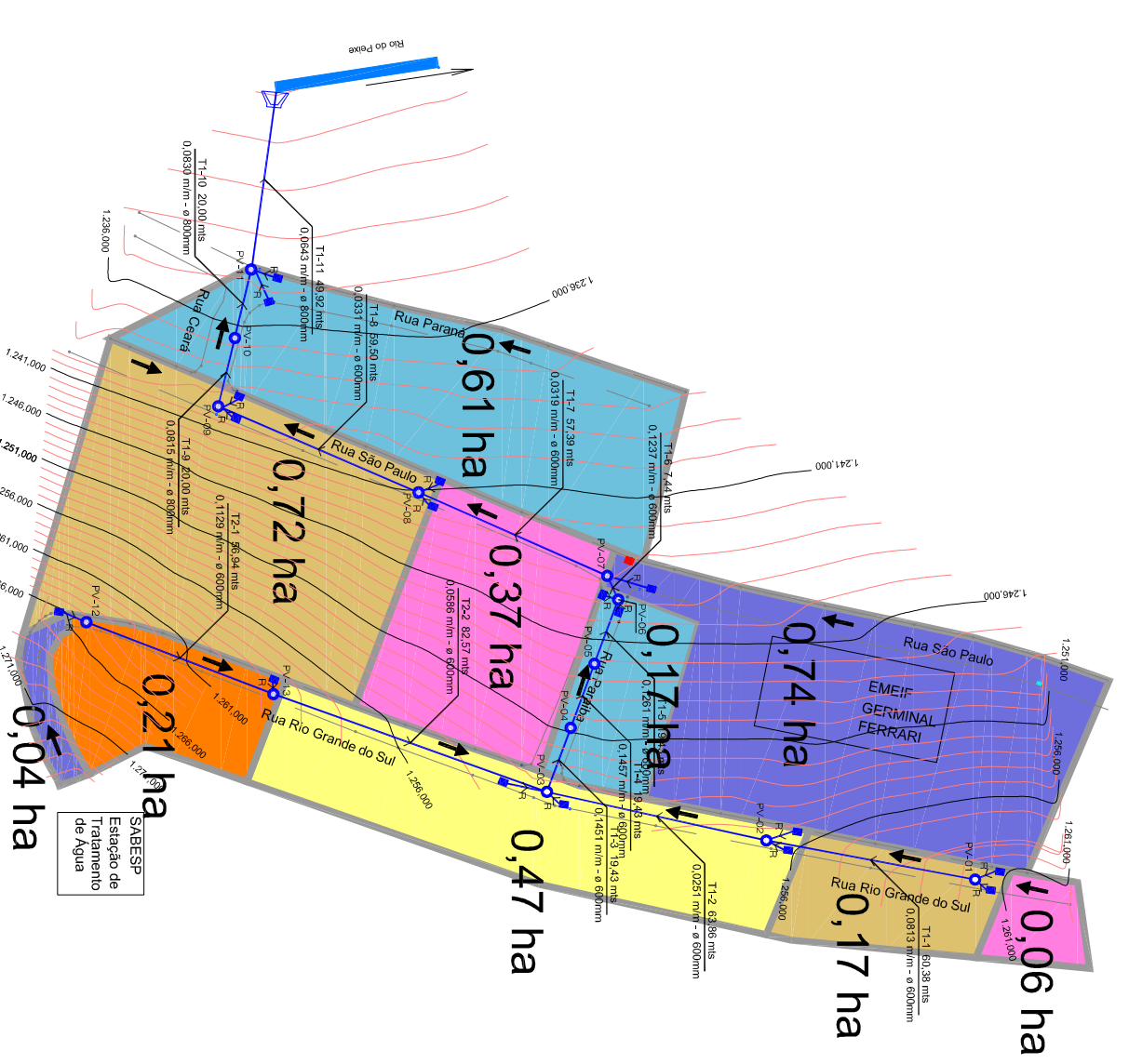
PLANTA BAIXA - SUB-BACIA DE CONTRIBUIÇÃO NO BAIRRO CAMPESTRINHO ESC: 1:2000
