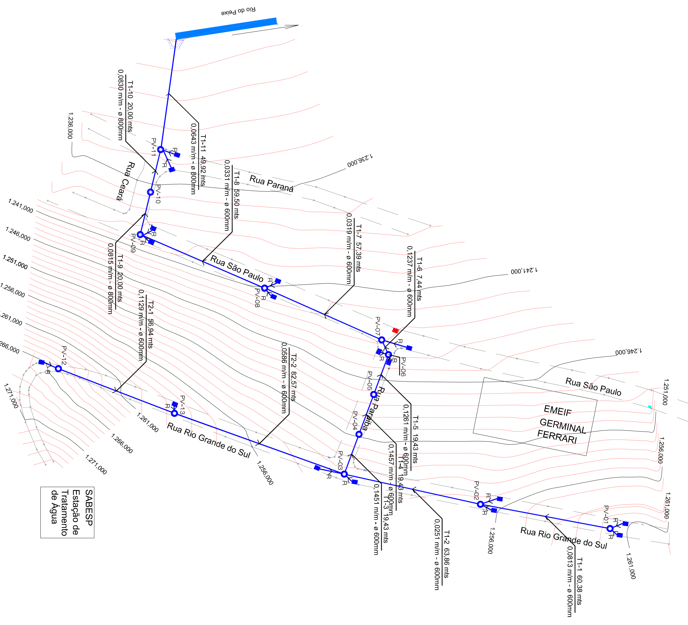
PLANTA BAIXA - RUAS DO BAIRRO CAMPESTRINHO ESC: 1:1000
