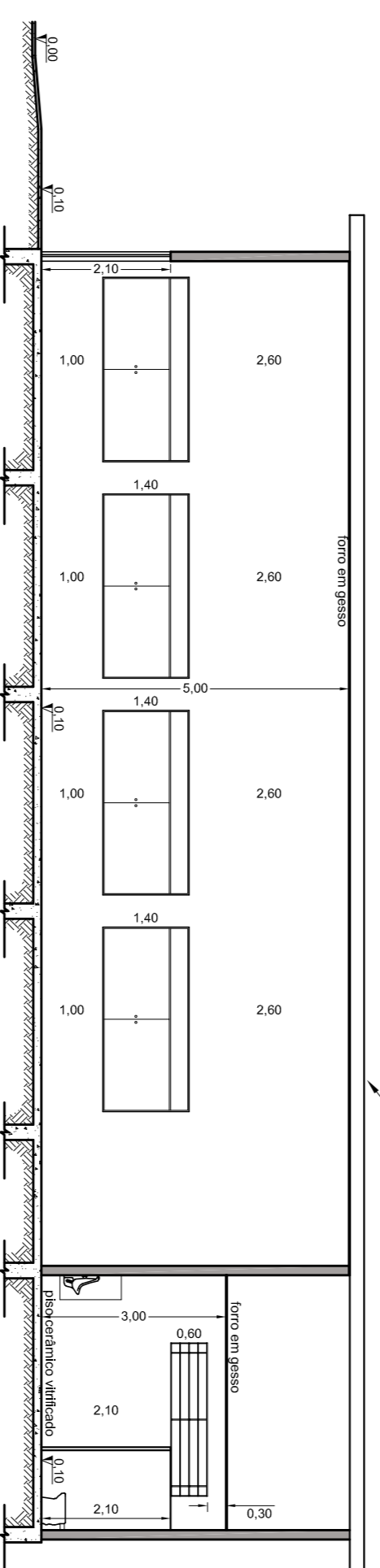
CORTE A-A ESC: 1/100
