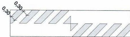
PINTURA DOS REDUTORES DE VELOCIDADE
