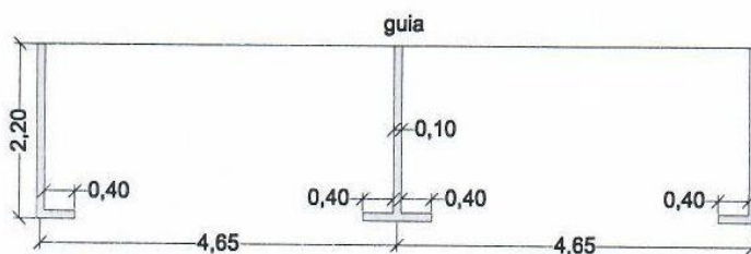
PINTURA DAS VAGAS PERPENDICULARES
