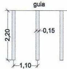
PINTURA DAS VAGAS DE MOTOS
