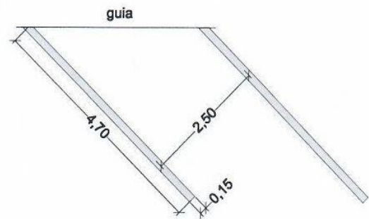
PINTURA DAS VAGAS 45°
