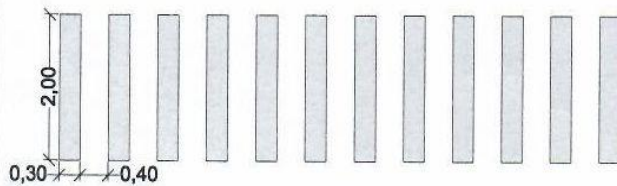
PINTURA DAS FAIXAS DE PEDESTRES
