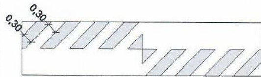
PINTURA DOS REDUTORES DE VELOCIDADE
