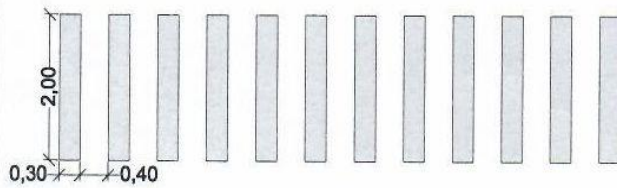
PINTURA DAS FAIXAS DE PEDESTRES PINTURA DAS FAIXAS ELEVADAS
